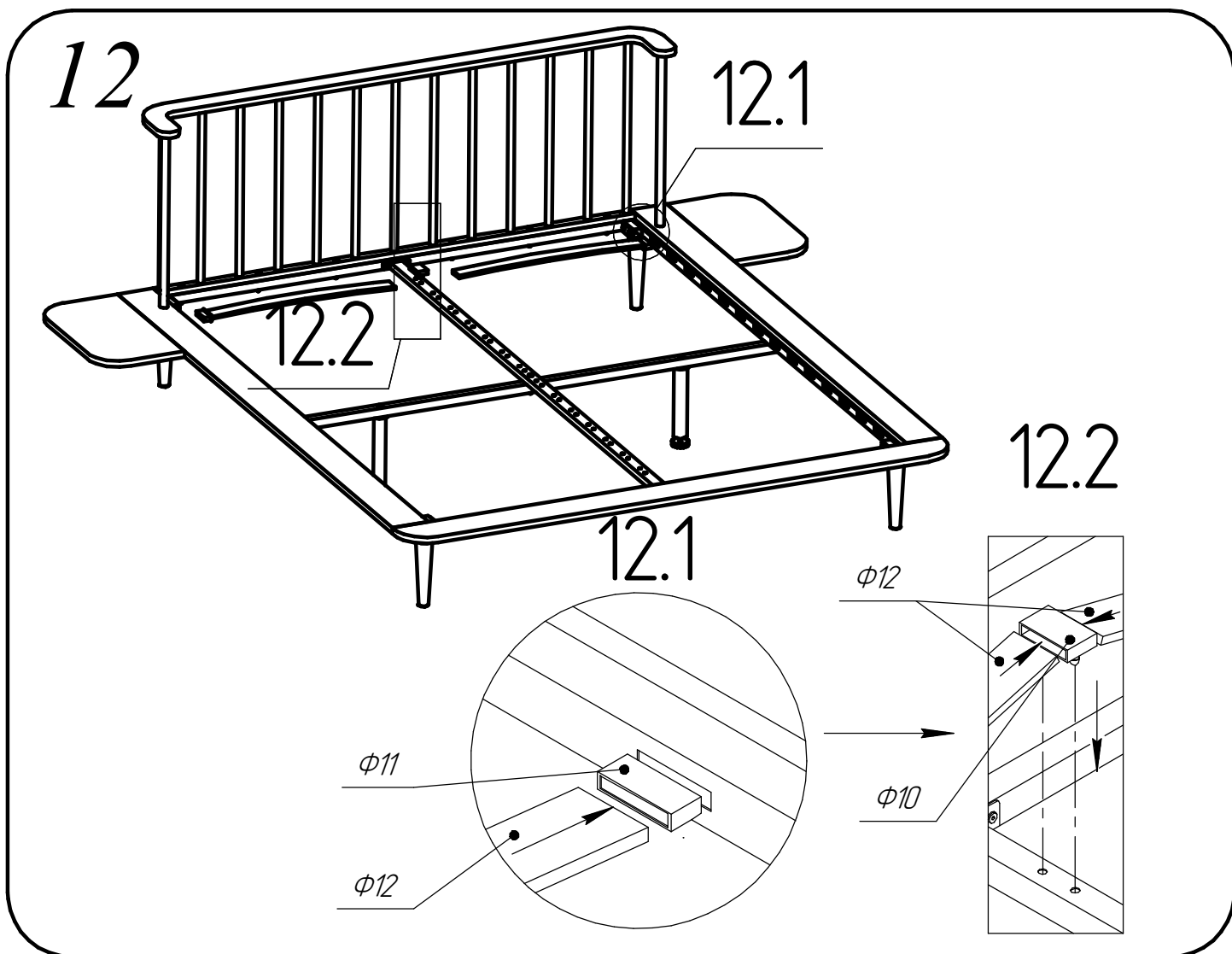
Инструкция по сборке кровати КМД-28 «Варна» («Барна») Версия 1 от 18.09.2023
